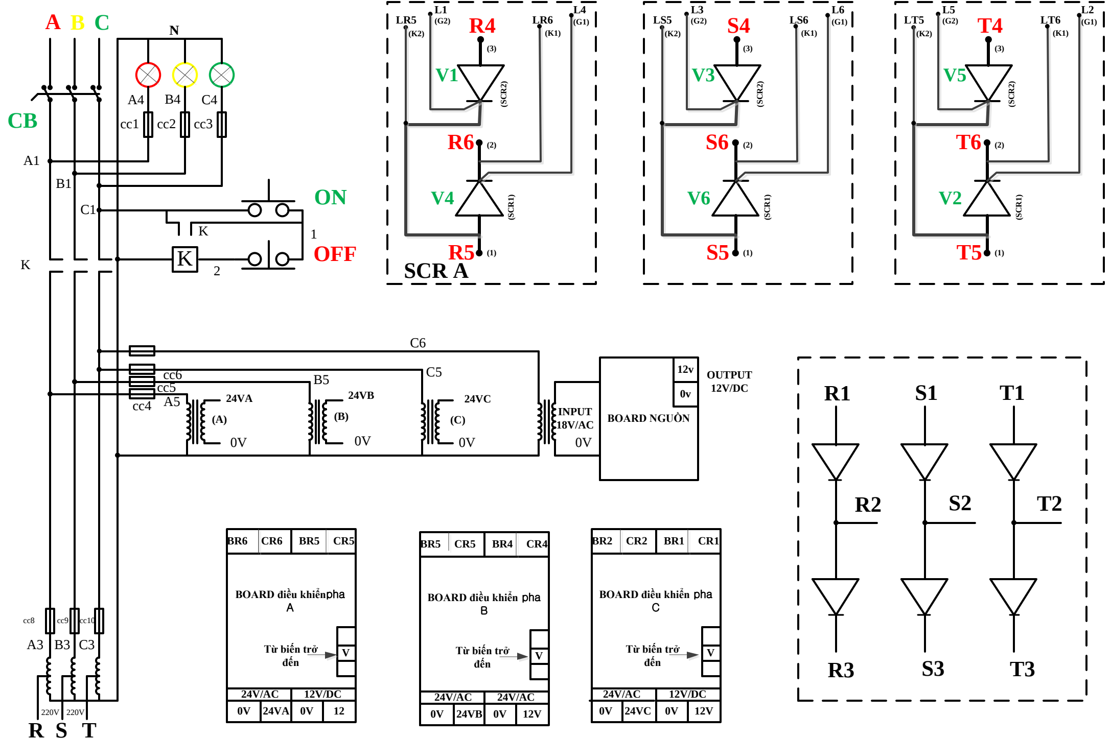
SƠ ĐỒ MẠCH TRONG TỦ THỰC TẬP ĐIỆN TỬ CÔNG SUẤT
